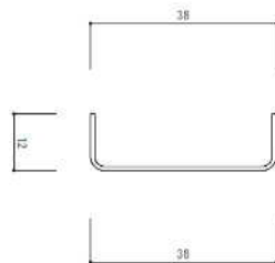
<図面>UCH 杉本)Cチャンネル 4m
