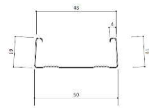
<図面> NTB2W 杉本)ダブルバー 3m
