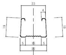
<図面> NTB1S 杉本)シングルバー 3m
