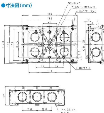
●寸法図(mm)
