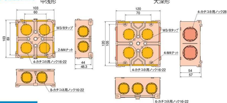
●寸法図 (mm)
