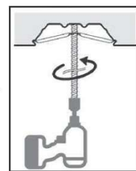
4 インパクトドライバー等を使用し吊りボルトをデッキに当たるまで締め付けて取付完了
