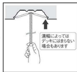
3 もう一方を押し上げる (デッキの溝にはまるとパチンと音がします)
