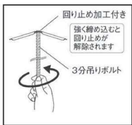
1 金具の先端まで吊りボルトを手でねじこむ
