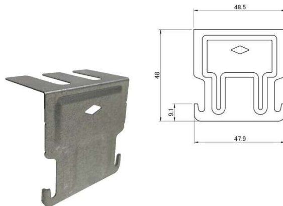
●寸法図(mm)
