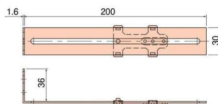
●寸法図(mm)
