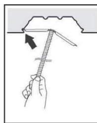
2 金具の片方の端をデッキの溝に合わせる
