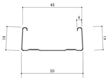
●寸法図(mm)
