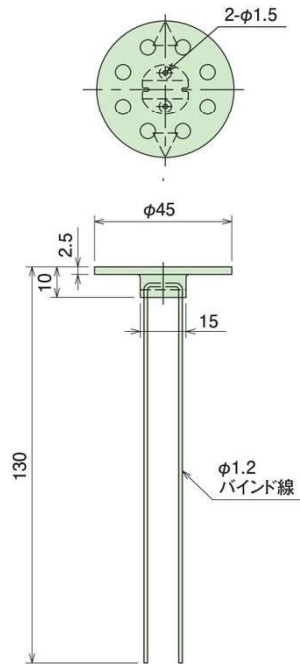
●寸法図 (mm)
