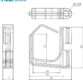
●寸法図 (mm)
