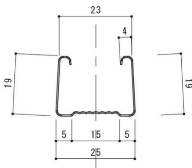
●寸法図(mm)
