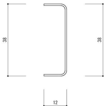
●寸法図(mm)
