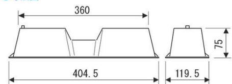
●寸法図
