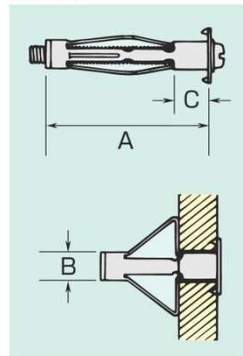
●寸法図
