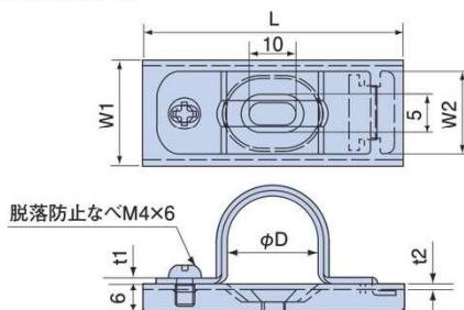
●寸法図(mm)
