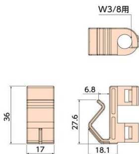
●寸法図 (mm)
