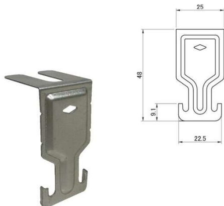
●寸法図(mm)
