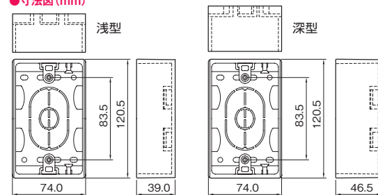
●寸法図 (mm)
