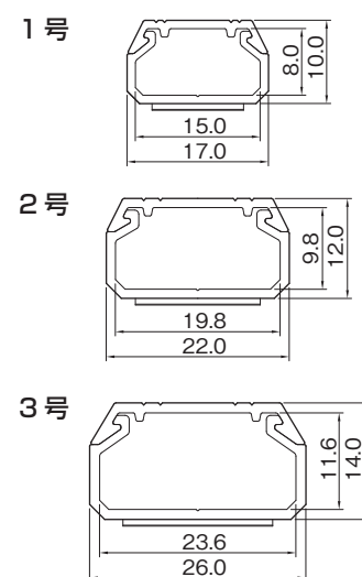
●断面図(mm)
