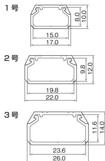
●断面図(mm)
