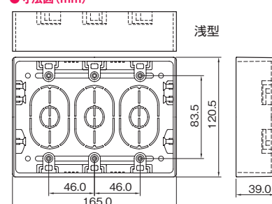
●寸法図 (mm)
