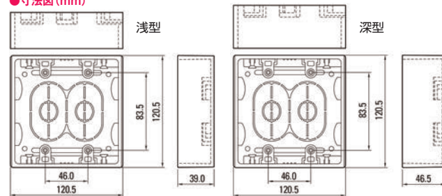
●寸法図 (mm)
