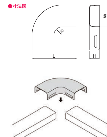
●寸法図
