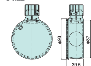
●寸法図
