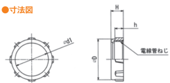
●寸法図
