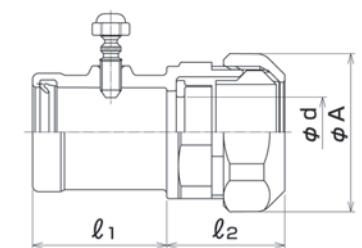
●寸法図
