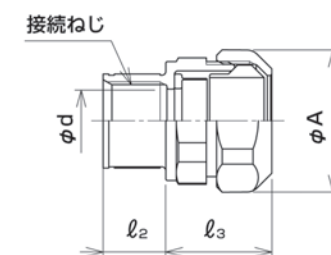
●寸法図
