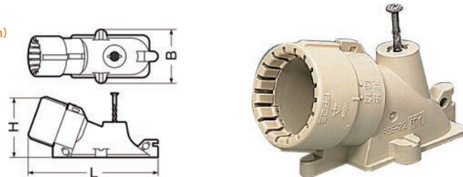
●寸法図 (mm)
