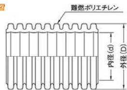
●寸法図
