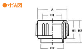
●寸法図
