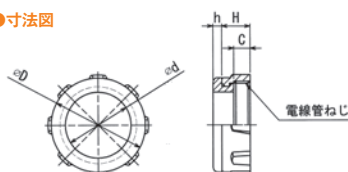
●寸法図
