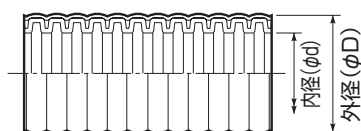
●寸法図(mm)
