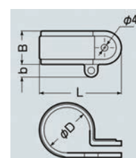
●寸法図
