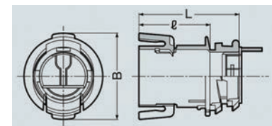
●寸法図(mm)
