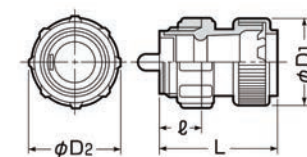
●寸法図(mm)
