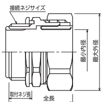
●寸法図
