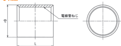
●寸法図
