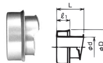
●寸法図
