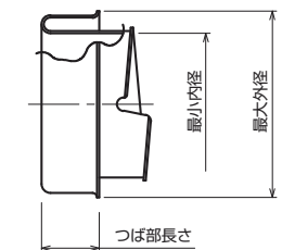
●寸法図
