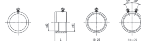
●寸法図
