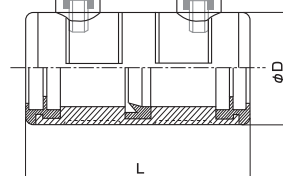
●寸法図
