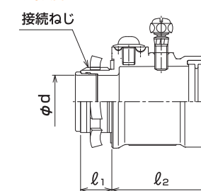
●寸法図
