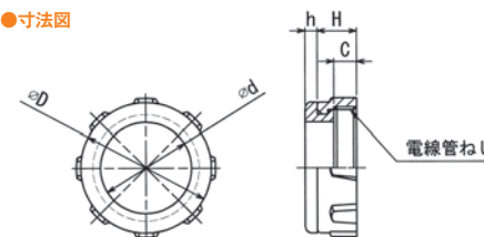
●寸法図
