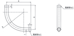
●寸法図
