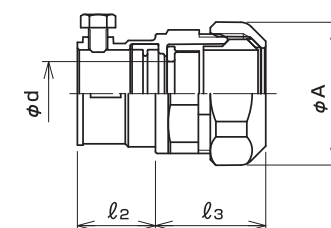
●寸法図
