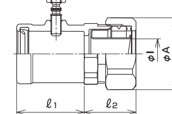
●寸法図
