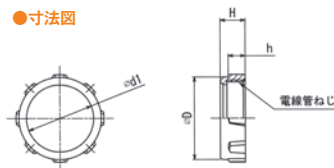
●寸法図
