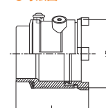
●寸法図
