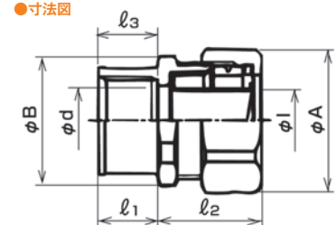
●寸法図
