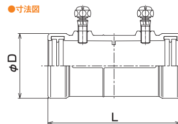
●寸法図
