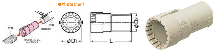
●寸法図 (mm)
