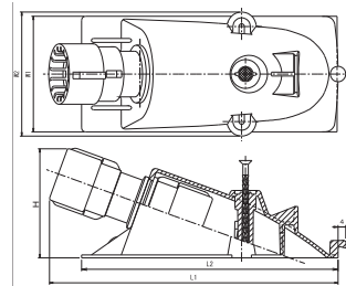
●寸法図(mm)
