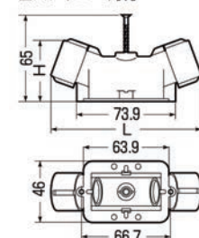
●寸法図(mm)
