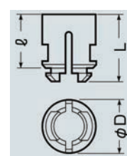
●寸法図
