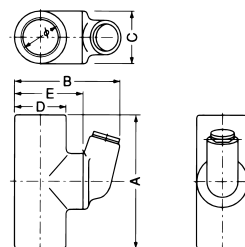
●寸法図
