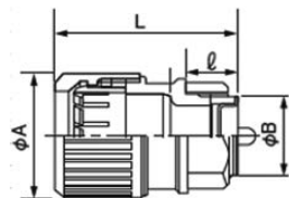
●寸法図
