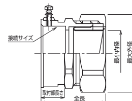
●寸法図
