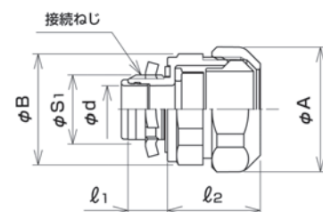
●寸法図
