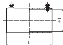
●寸法図
