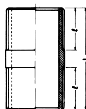
●寸法図
