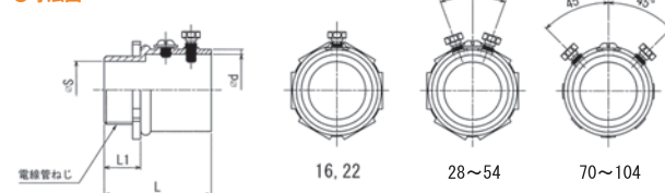
●寸法図
