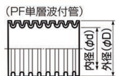
●寸法図(mm)
