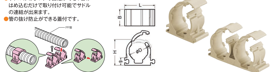
●寸法図 (mm)
