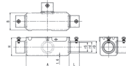
●寸法図
