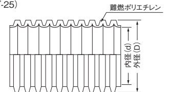
●寸法図 （タイプ-25）
