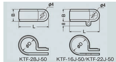
●寸法図 (mm)
