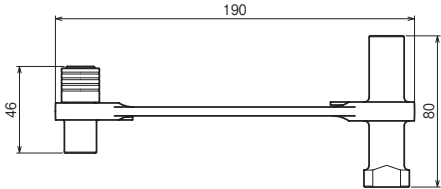
●寸法図
