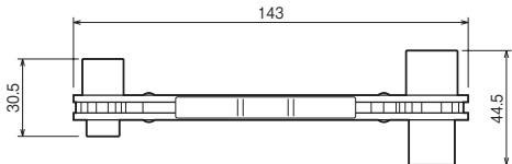
●寸法図
