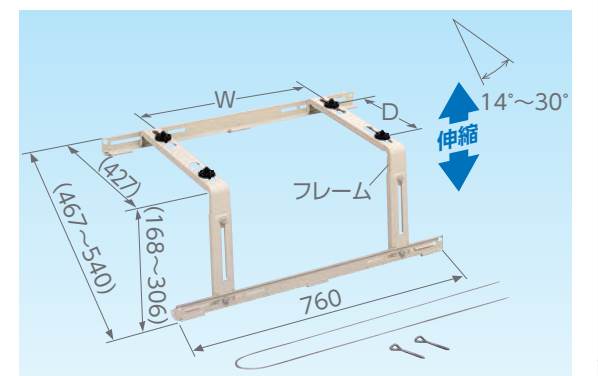
フレームを逆にした組み立て方
