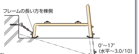
フレームを逆にした組み立て方
