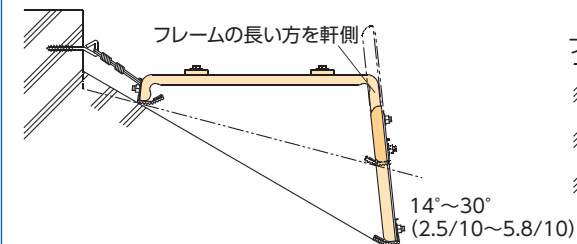
通常の組み立て方
