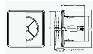
●寸法図
