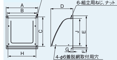
●寸法図
