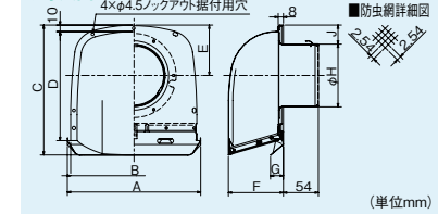
●寸法図
