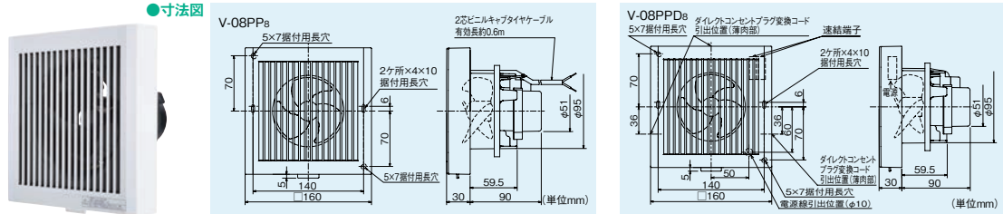
●寸法図
