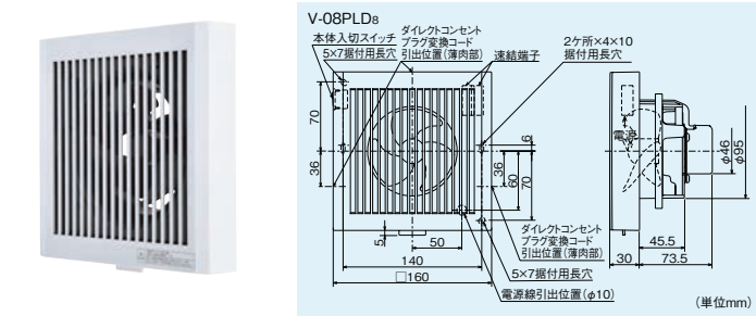
●寸法図
