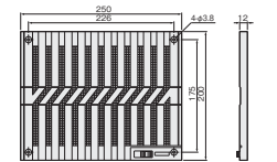
●詳細図
