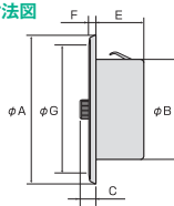
●寸法図
