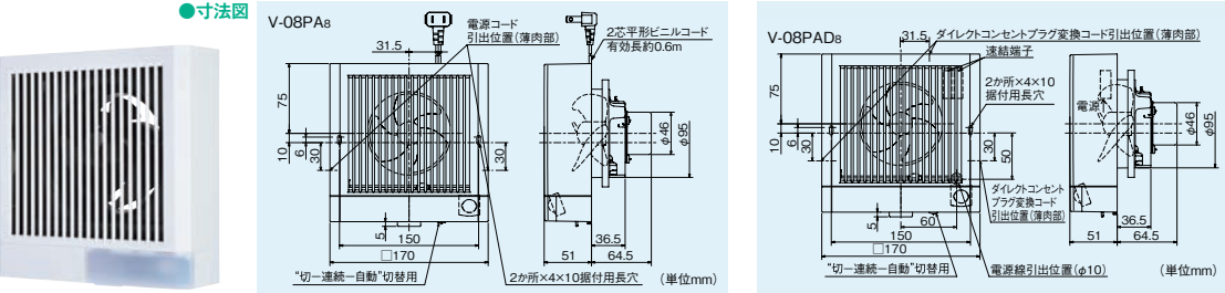
●寸法図
