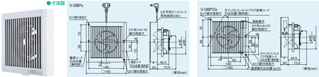
●寸法図
