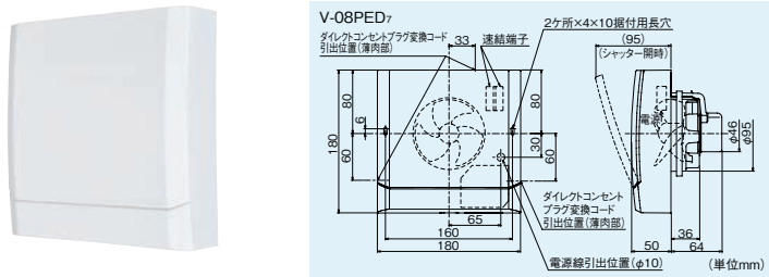
●寸法図
