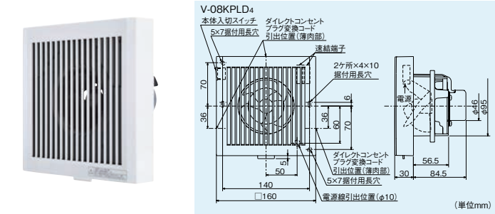
●寸法図
