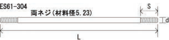
●寸法図
