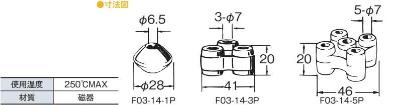
●寸法図
