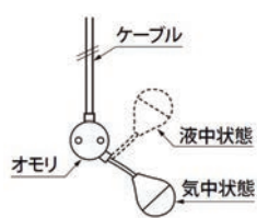
●状態図
