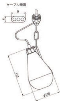
●寸法図
