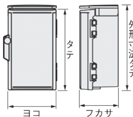
●寸法図
