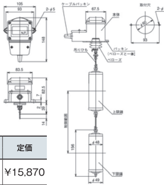
●寸法図
