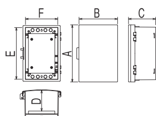
●寸法図
