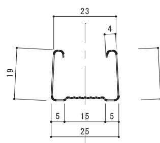
●寸法図(mm)
