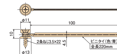
●寸法図 (mm)
