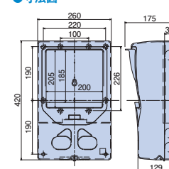
●寸法図
