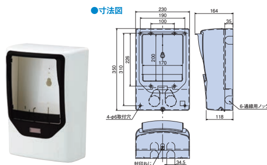
●寸法図
