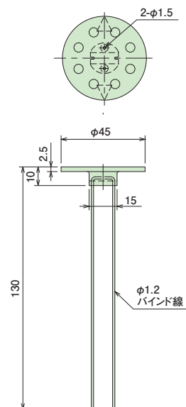
●寸法図 (mm)
