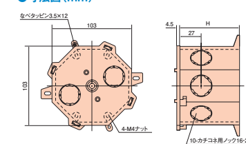
●寸法図 (mm)
