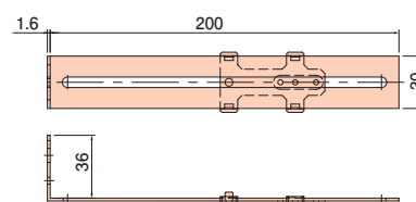
●寸法図 (mm)
