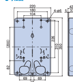
●寸法図
