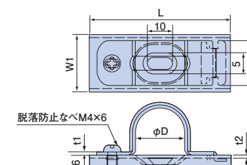
●寸法図 (mm)
