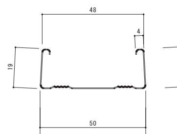
●寸法図(mm)
