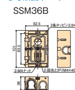
●寸法図 (mm)
