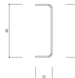
●寸法図(mm)
