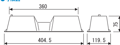
●寸法図
