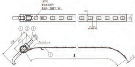
●寸法図
