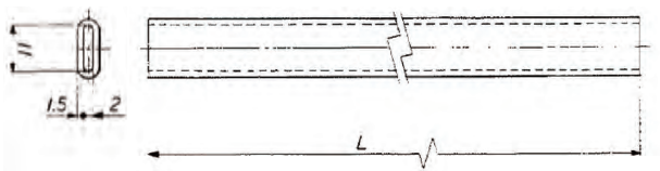
●寸法図
