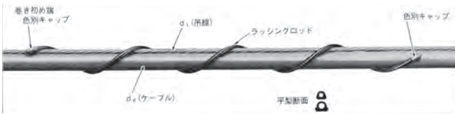
●施工例
