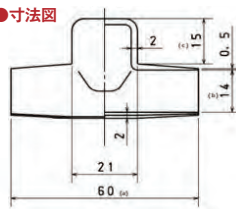
●寸法図
