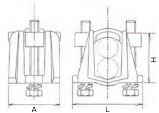
●寸法図
