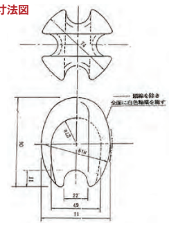
●寸法図
