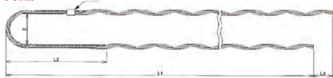
●寸法図
