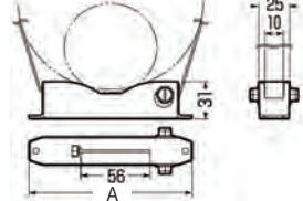
●寸法図
