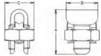
●寸法図
