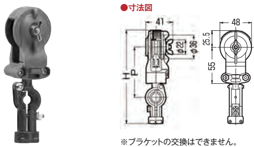
●寸法図
