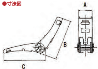
●寸法図
