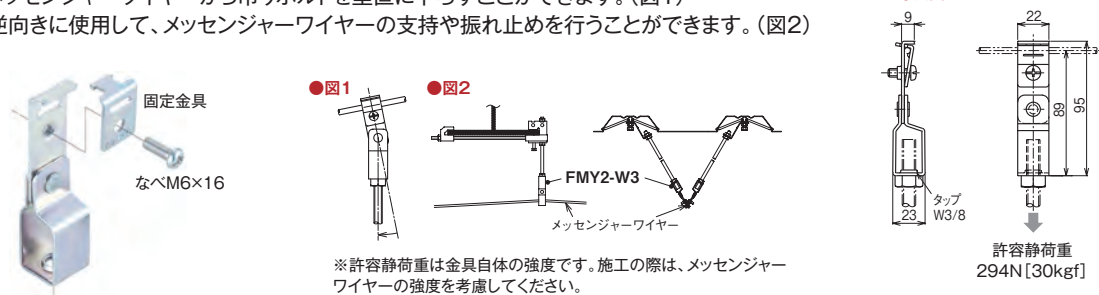
●寸法図
