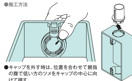
●施工方法
