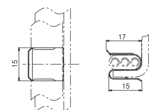
●寸法図 (mm)
