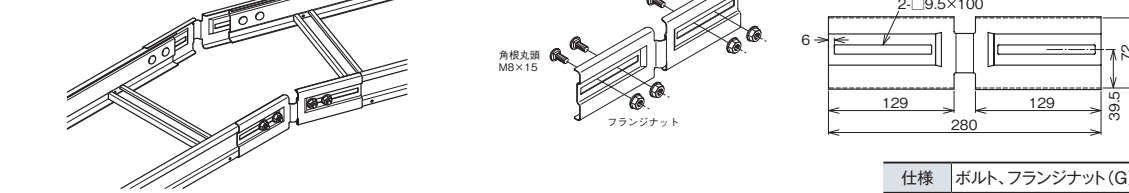
●寸法図 (mm)
