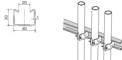
●寸法図 (mm)
