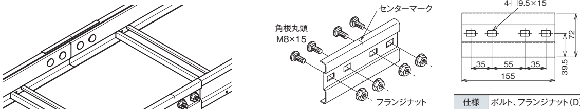
●寸法図 (mm)
