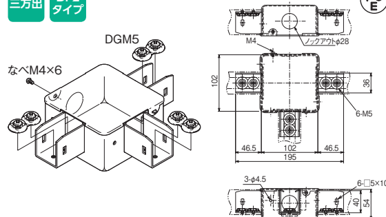
●寸法図 (mm)
