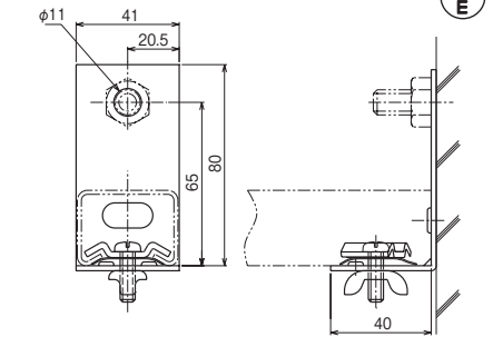
●寸法図 (mm)
