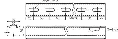
●寸法図 (mm)
