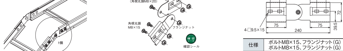
●寸法図 (mm)
