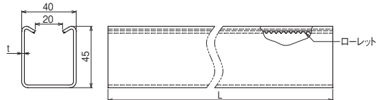
●寸法図 (mm)
