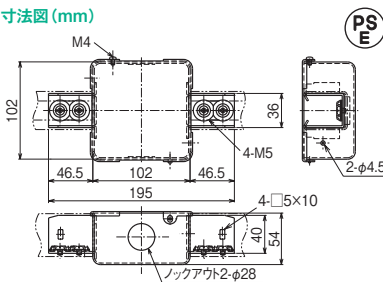
●寸法図 (mm)
