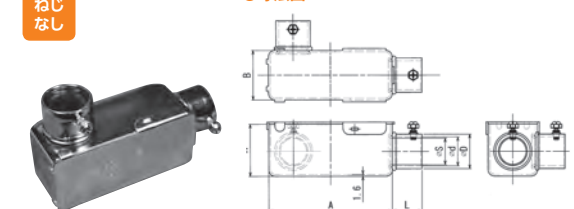
●寸法図
