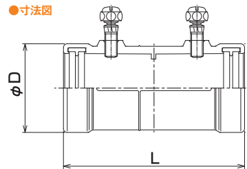
●寸法図
