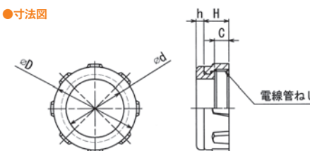
●寸法図
