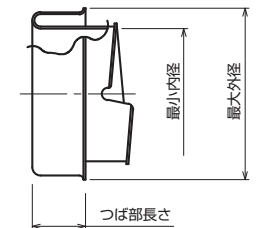
●寸法図
