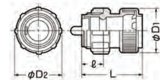
●寸法図(mm)
