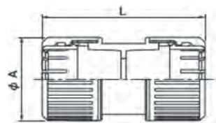
●寸法図
