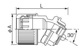
●寸法図(mm)
