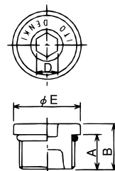
●寸法図
