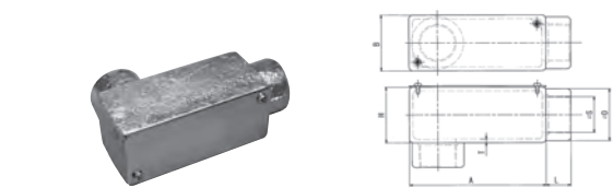
●寸法図
