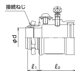
●寸法図
