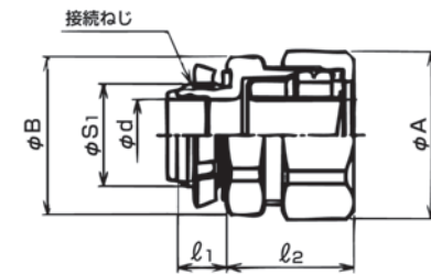
●寸法図
