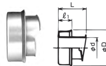
●寸法図
