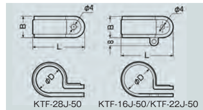
●寸法図 (mm)
