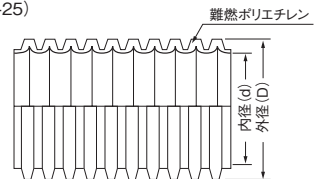
●寸法図 （タイプ-25）
