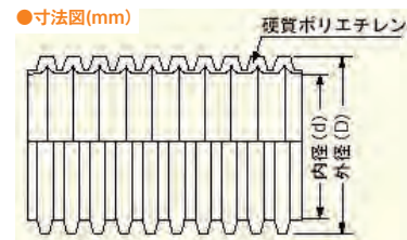
●寸法図(mm)
