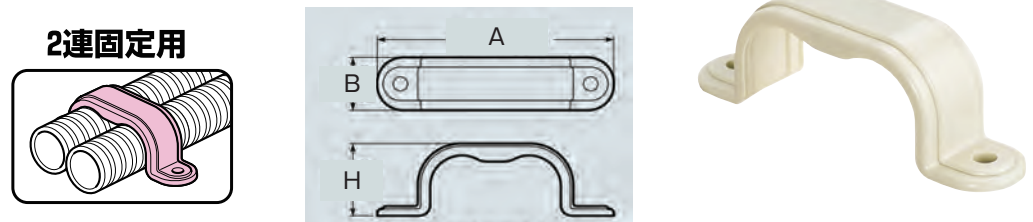
●寸法図 (mm)
