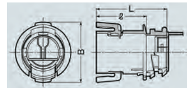
●寸法図(mm)
