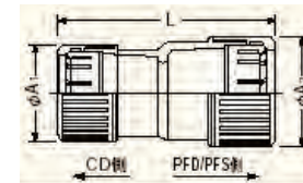
●寸法図(mm)
