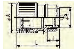
●寸法図(mm)
