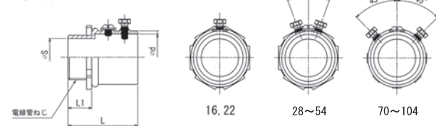
●寸法図
