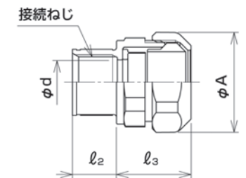
●寸法図
