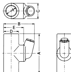
●寸法図
