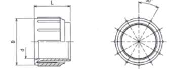
●寸法図
