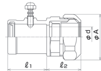
●寸法図
