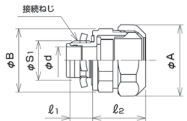
●寸法図
