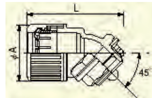
●寸法図(mm)
