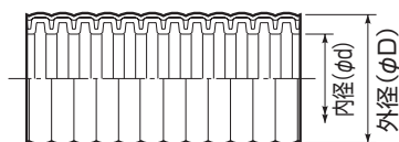
●寸法図(mm)
