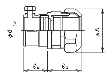
●寸法図
