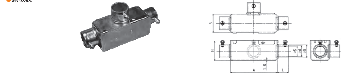
●寸法図
