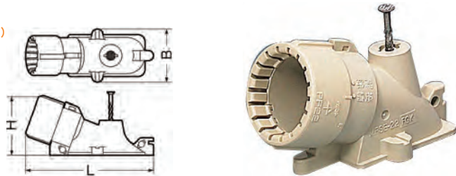
●寸法図 (mm)
