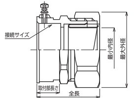
●寸法図
