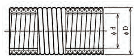
●寸法図
