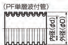
●寸法図(mm)
