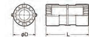
●寸法図(mm)
