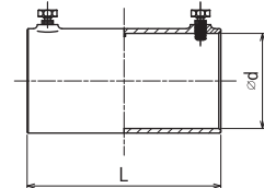
●寸法図
