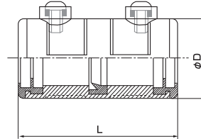
●寸法図
