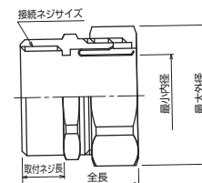
●寸法図
