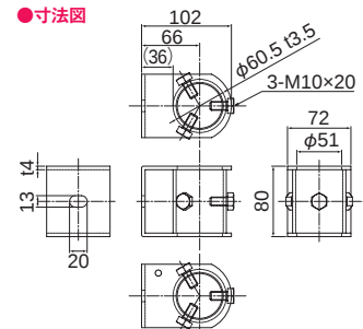
●寸法図
