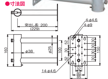
●寸法図
