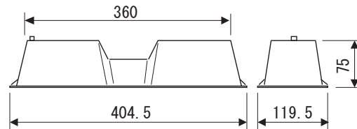
●寸法図
