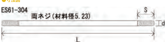
●寸法図
