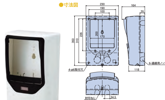
●寸法図
