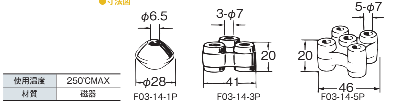
●寸法図
