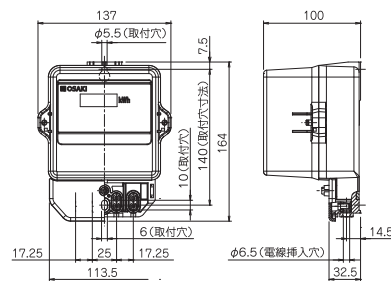
●寸法図
