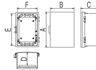
●寸法図
