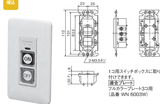
●寸法図
