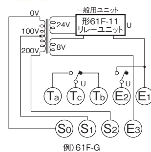
●内部配線図
