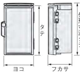
●寸法図
