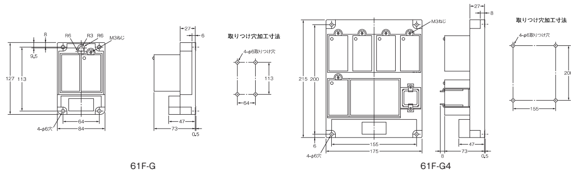
●寸法図
