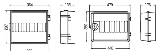
●寸法図
