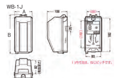
●寸法図
