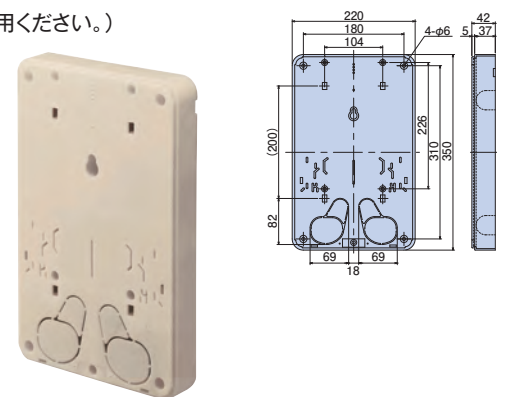
●寸法図
