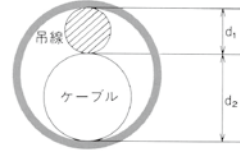
●寸法図
