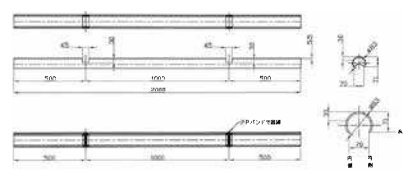
●寸法図
