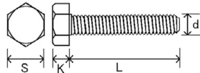
●寸法図
