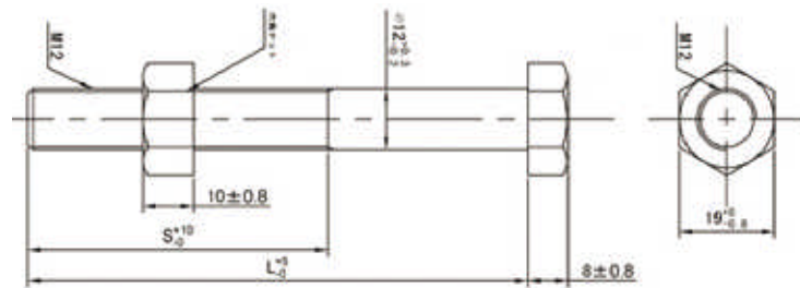
●寸法図
