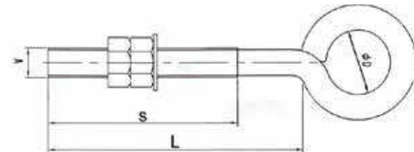
●寸法図
