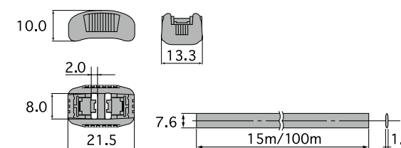
● 寸法図
