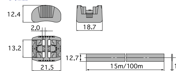
● 寸法図
