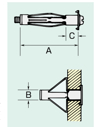
●寸法図
