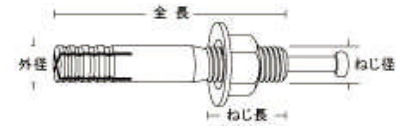
●寸法図
