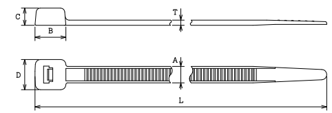
●寸法図
