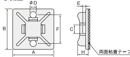
● 寸法図
