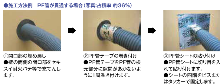
●施工方法例 PF管が貫通する場合(写真:占積率 約36%)
