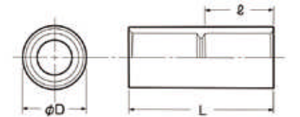
●寸法図
