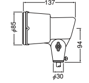
●寸法図
