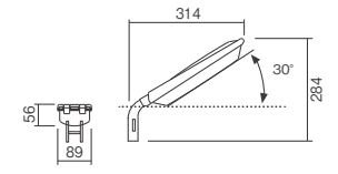
●寸法図
