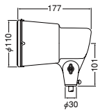
●寸法図
