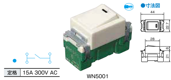
定格 15A 300V AC
