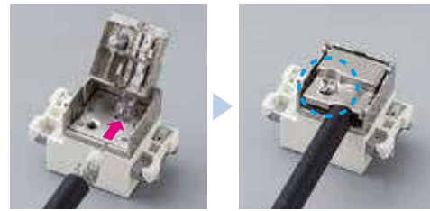
「らくらく端子」に心線を差し込み、金具をネジ止め(1カ所)するだけ。
