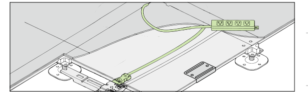
接地2P15A125V 接地2P15A125V 抜け止め
