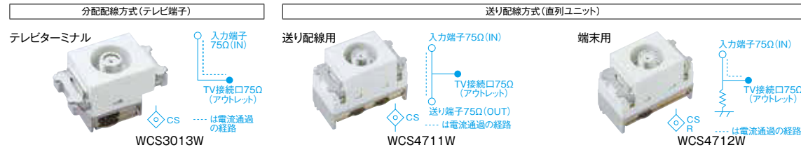
「らくらく端子」に心線を差し込み、金具をネジ止め(1カ所)するだけ。
