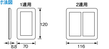
2連にてスイッチコンセントを組み合わせる場合はスイッチ+コンセントプレートをご使用ください。
