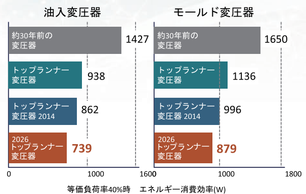
エネルギー消費効率の比較 (三相 50Hz 300kVA)
