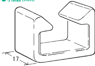
●寸法図 (mm)
