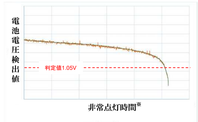
マイコンの電池電圧検出値(対策後)
