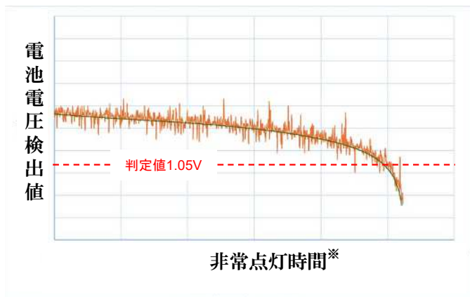
マイコンの電池電圧検出値(対策前)
