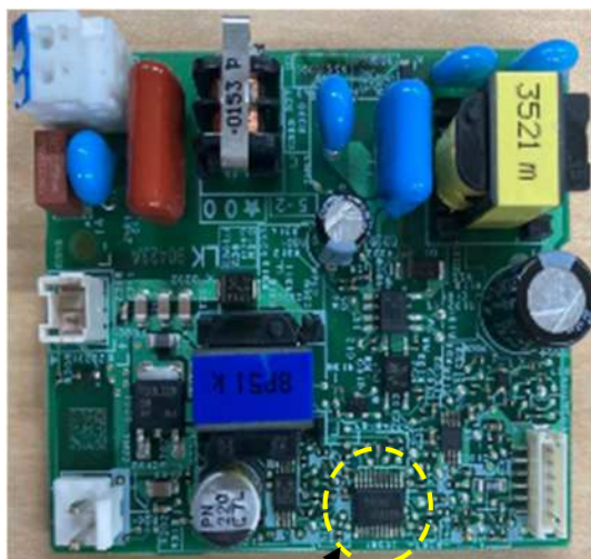
非常灯制御ブロック基板
